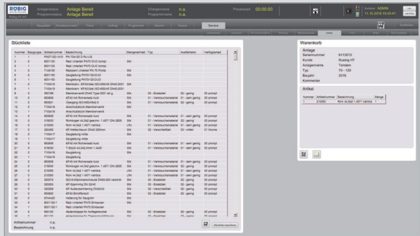
Der Anlagenzustand wird kontinuierlich dem Bediener visualisiert, wie z. B. eine Wartungsanzeige für auszuwechselnde, schadhafte Komponenten mit allen vakanten Zusatzinformationen und einem Warenkorb für die Bestellmöglichkeit von Ersatzteilen.
